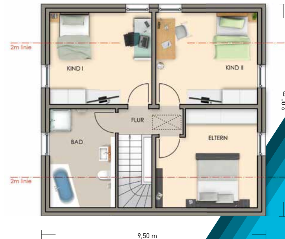
1:100 Dachgeschoss
